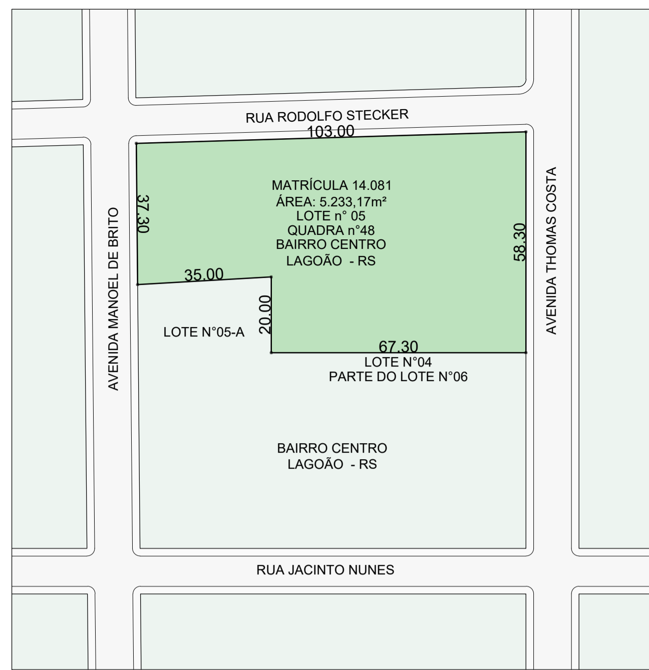
N PLANTA DE SITUAÇÃO ESC: 1 / 1000
