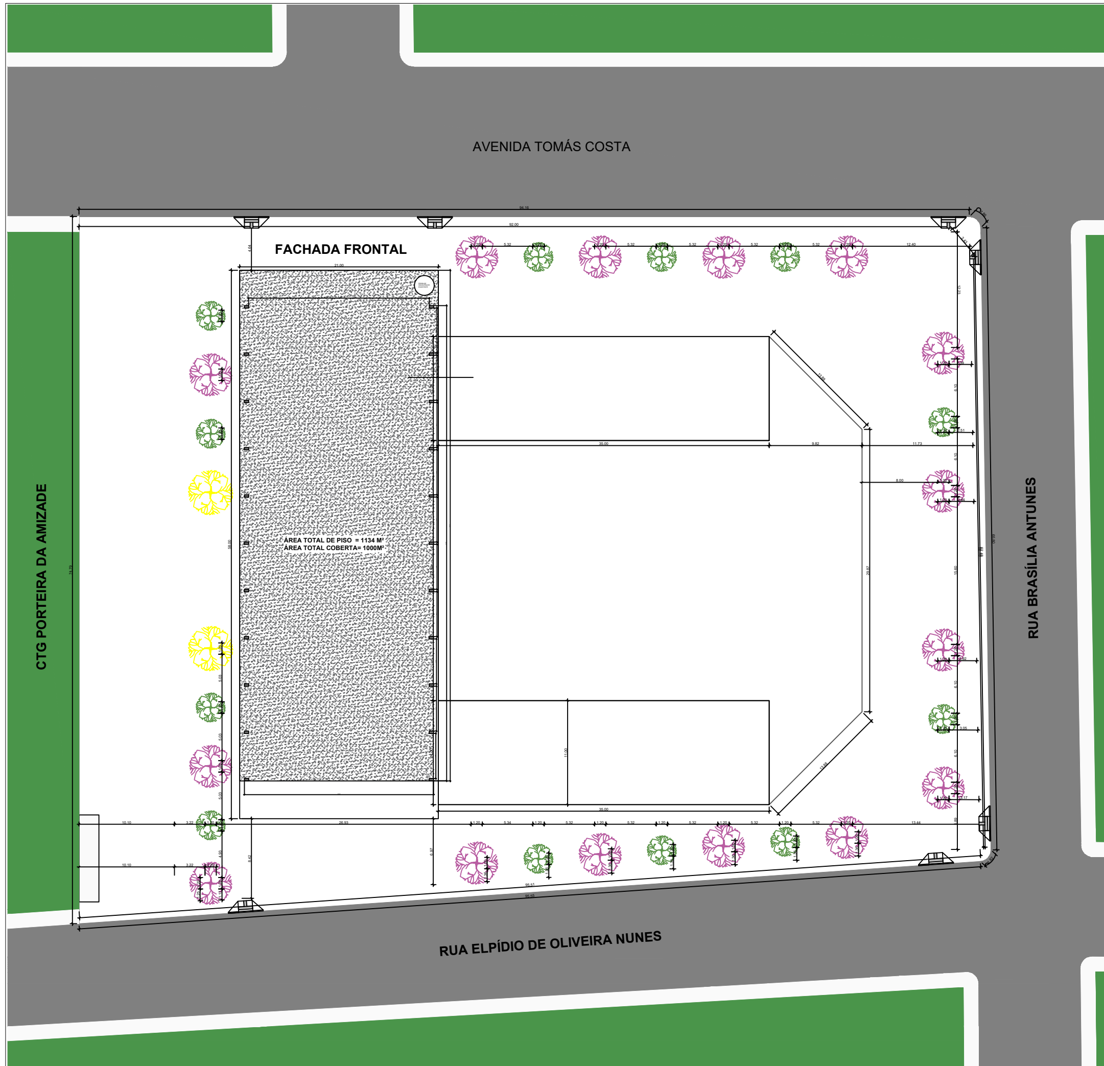
N PLANTA DE LOCALIZAÇÃO ESC: 1 / 200
