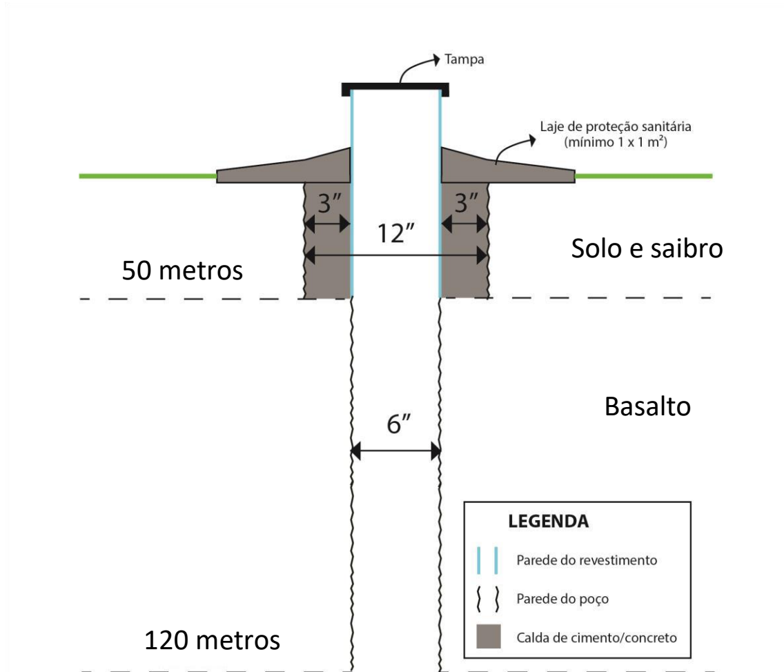
Figura 3: Perfil Geológico e Projeto Construtivo Básico do poço tubular.
