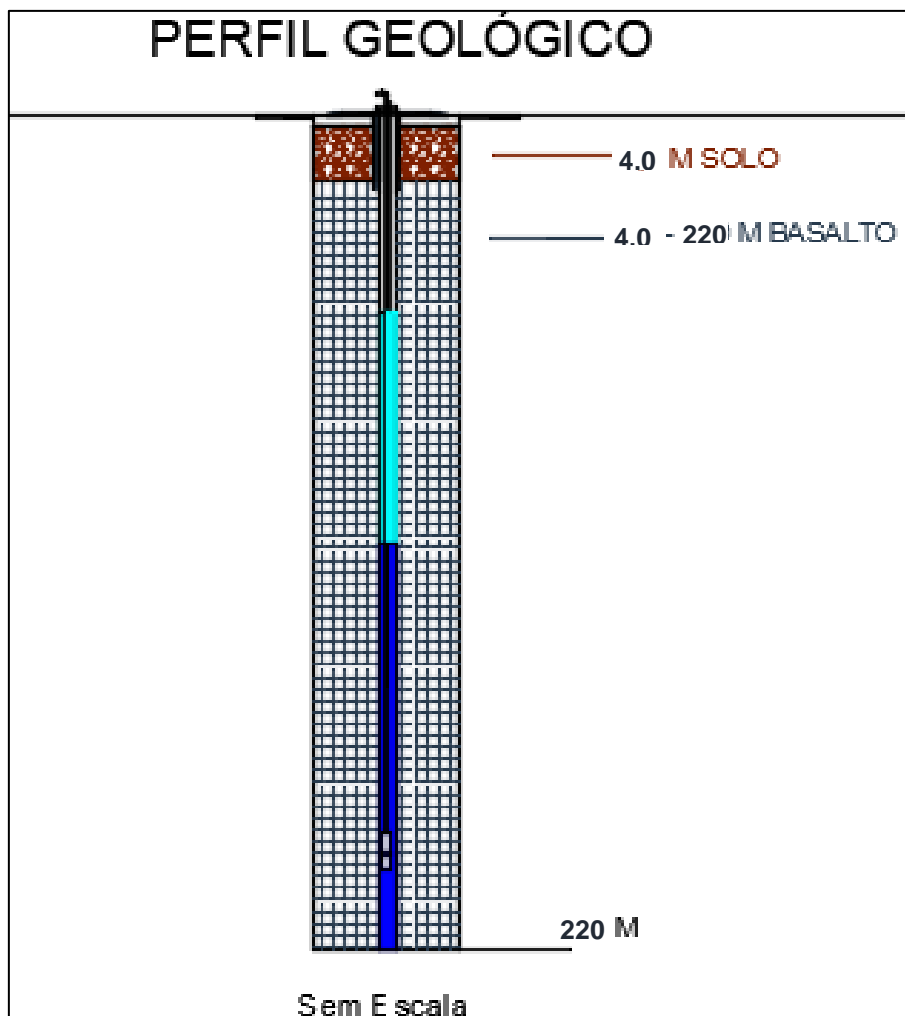
Figura 7 - Perfil geológico previsto no local de instalação do poço
