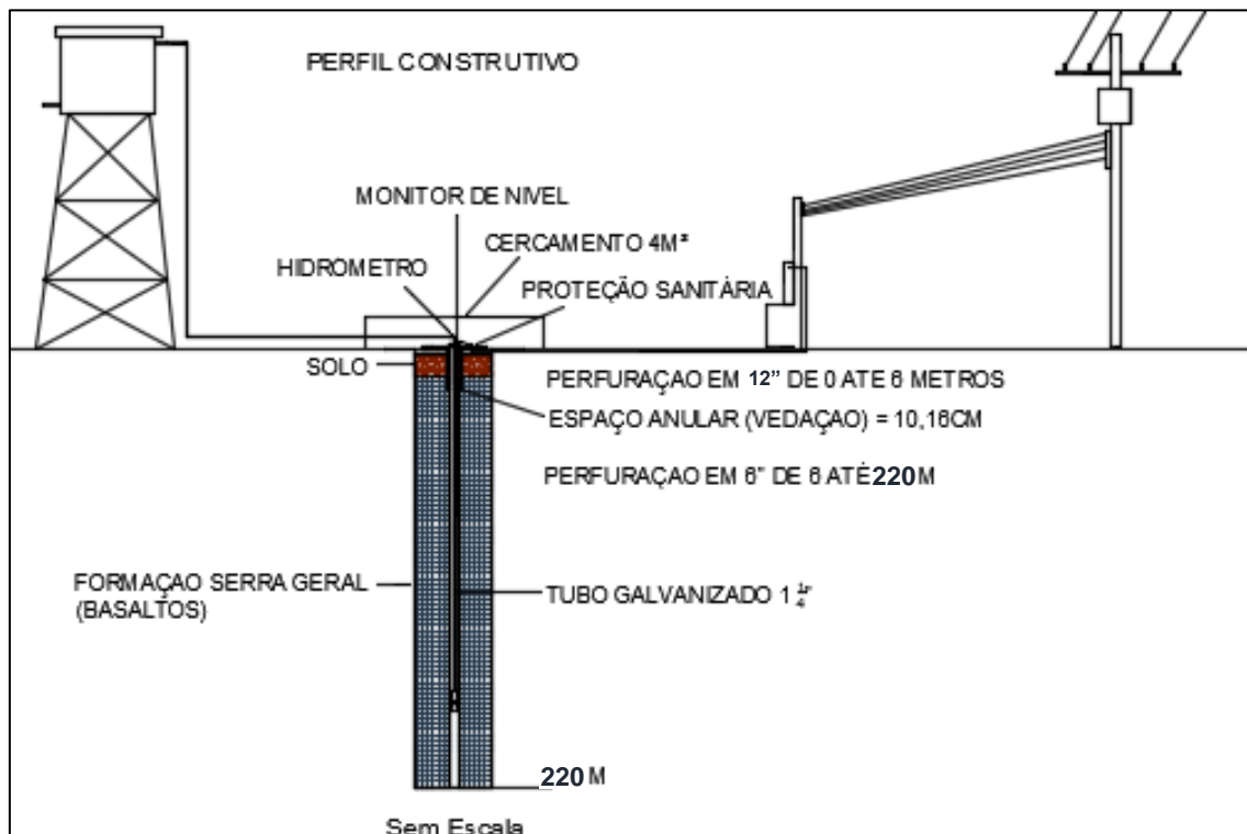
Figura 8 - Perfil Construtivo do Poço
